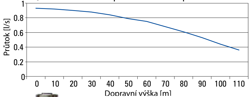
Q-H charakteristika pro nerezové čerpadlo MORAVA
